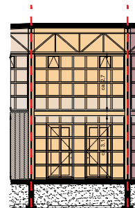
Doorsnede B-B
